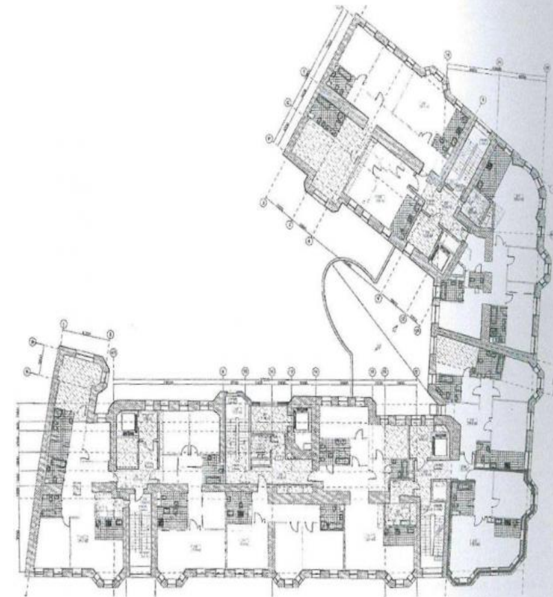
Предварительный (проектный) план второго этажа Многоквартирного жилого дома
