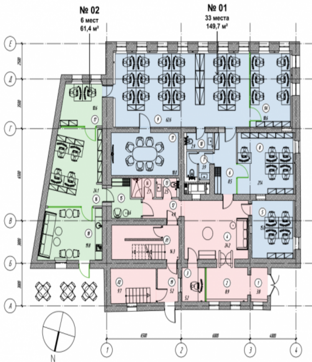
План расстановки мебели 1 этаж
