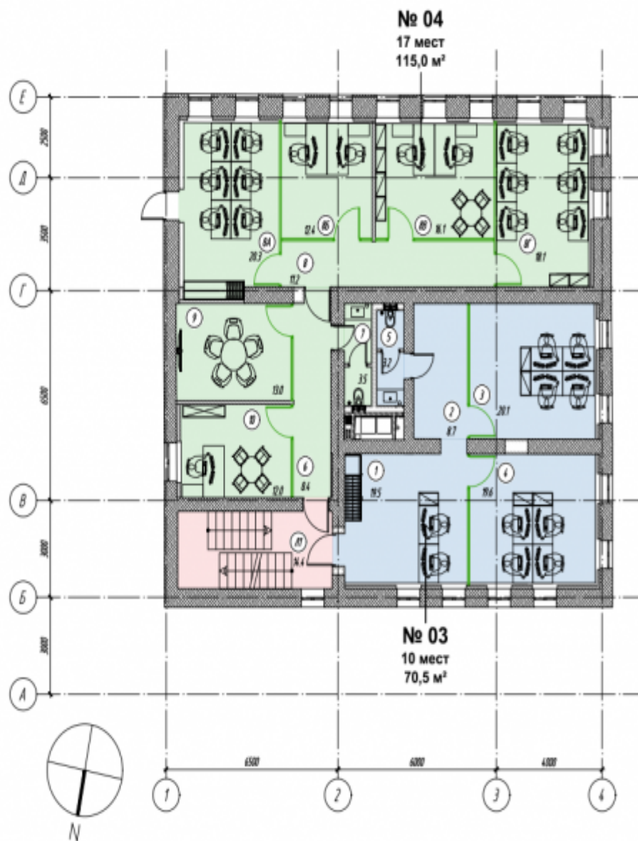
План расстановки мебели, 2 этаж
