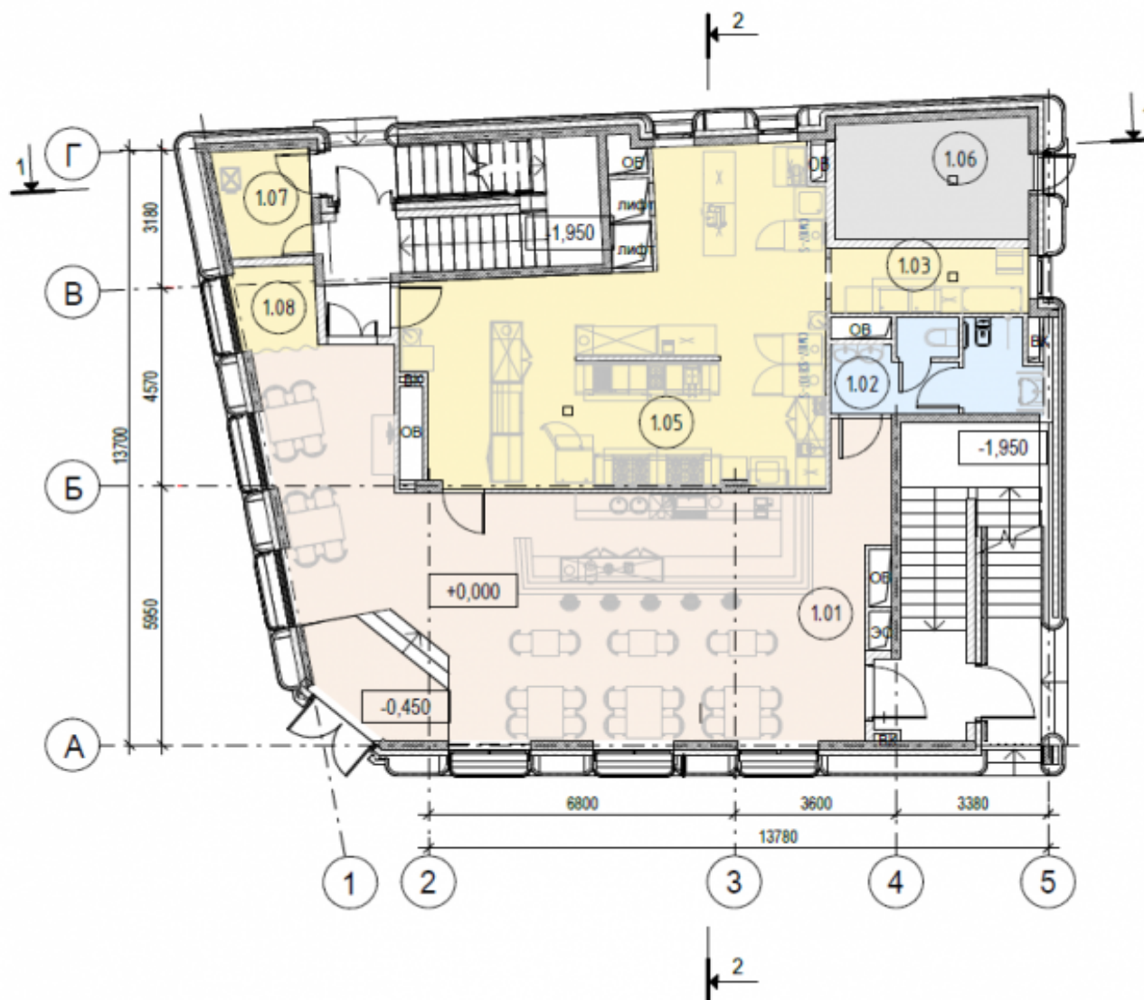
Схема плана 1-го этажа (на основе М 1:200)
