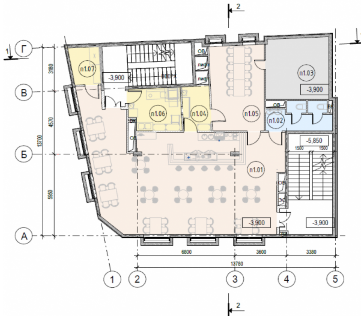
Схема плана цокольного этажа (на основе М 1:200)
