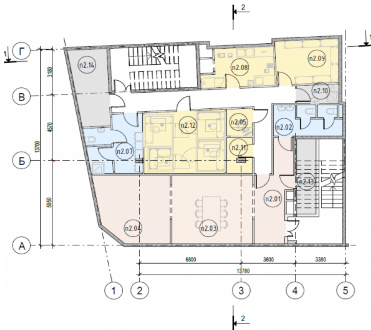
Схема плана подвального этажа (на основе М 1:200)
