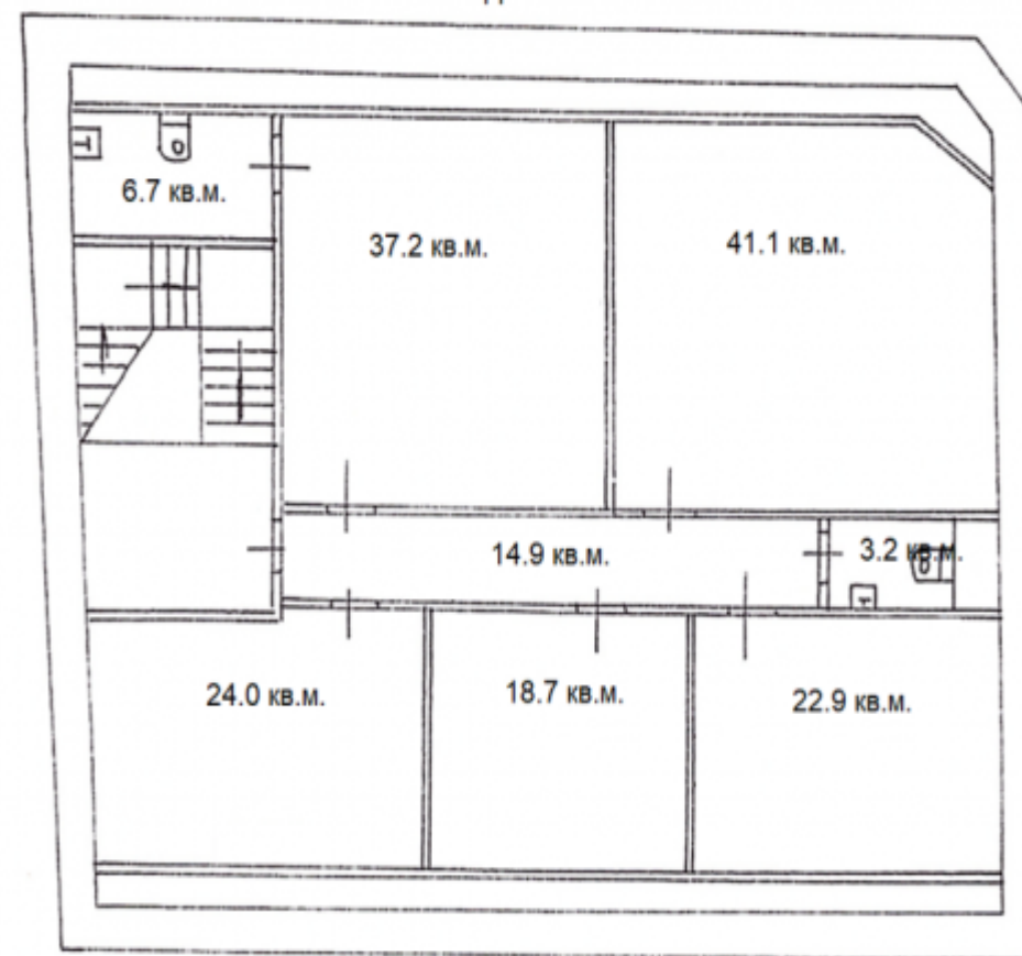
ЧЕРДАК/ ЭТАЖ 3
